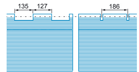
Détail charnière repère 1 et 2
