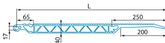
Profil de fermeture latéral (proposé en option) Référence: 390.00.019
